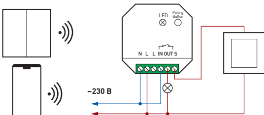
Рис. 1. Пример схемы подключения релейного модуля TY-701-72-DRI-DRO-PS-IN к светодиодным источникам и проводному выключателю
