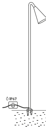
Рис. 3. Установка светильника на твердую поверхность
