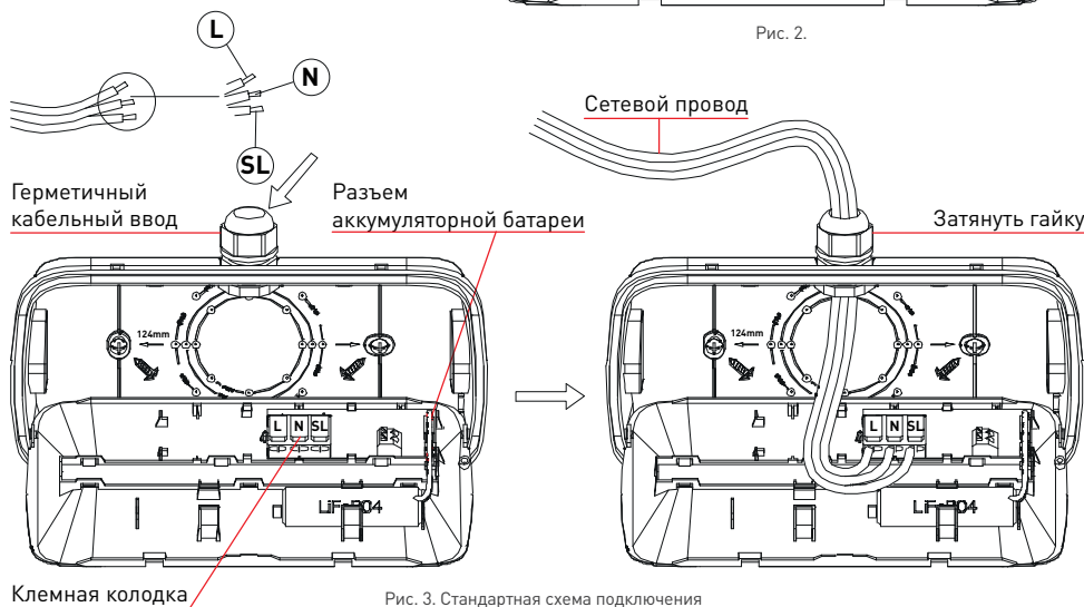
Рис. 3. Стандартная схема подключения
