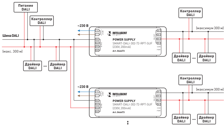
Рис. 3. Схема подключения шины DALI вертикальное размещение
