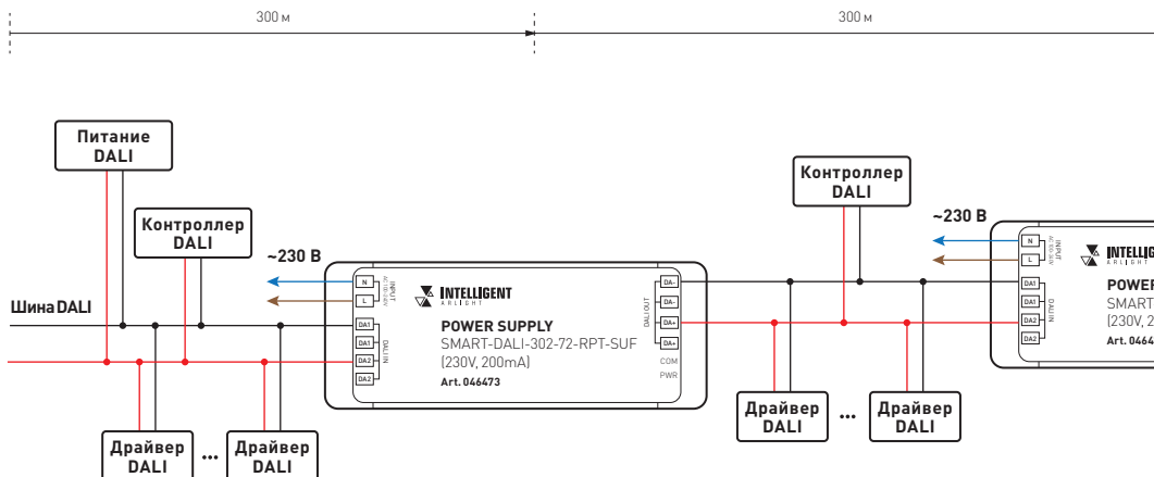
Рис. 2. Схема подключения шины DALI горизонтальное размещение
