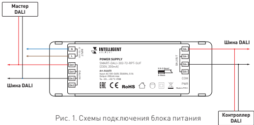
Рис. 1. Схемы подключения блока питания
