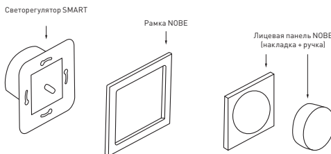
Рис. 5. Монтаж светорегулятора
