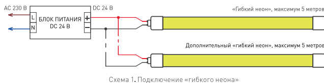
Схема 1. Подключение «гибкого неона»
