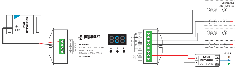
Четыре светодиодных светильника 350–1200 мА
