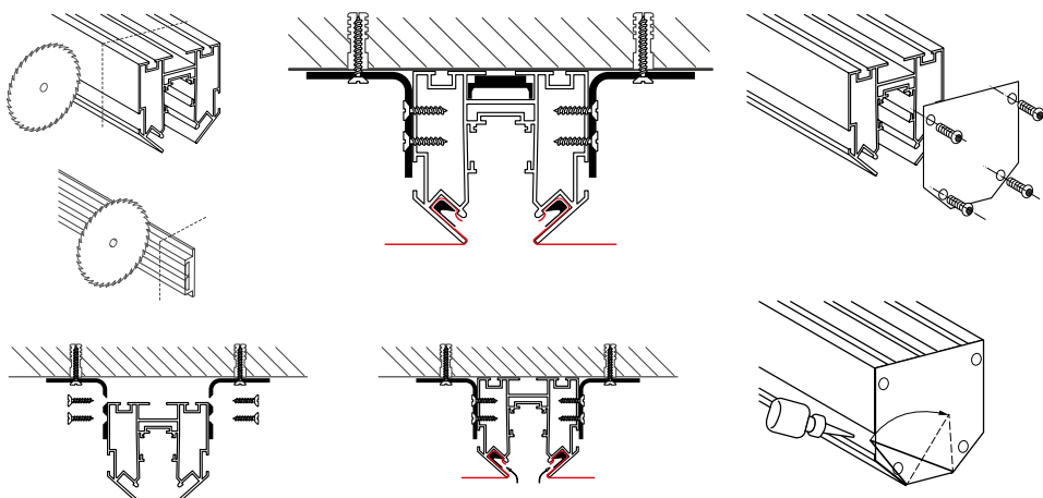
Рис. 2. Установка трека и монтаж натяжного потолка
