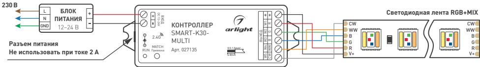
Рисунок 1. Схема подключения контроллера
