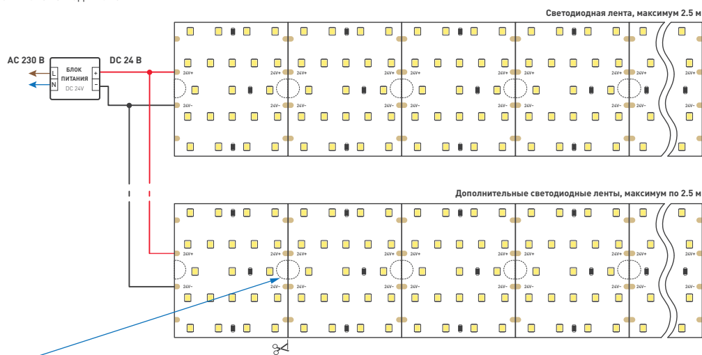
Схема 1. Подключение нескольких светодиодных лент
