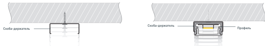
Рис. 2. Установка профиля
